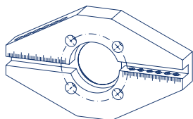
Porte-outil ID 58 - OD 219,1 mm 091505605
