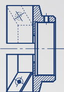
WP-Porte-outils 30° ID 40 - OD 78 mm 091501103
