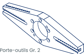
Porte-outil ID 280 - OD 711 mm 091503168
