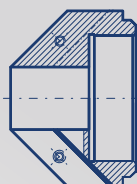
WP-Porte-outils 0° ID 25 - OD 66 mm 010007079
