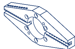
Porte-outils Gr. 1 ID 100 - OD 330 mm 091506031
