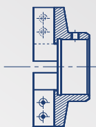
WP-Porte-outils 0° ID 40 - OD 104 mm 091501104
