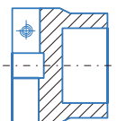
091504432 Porte-outils de la gamme 0° ID 10 - OD 38 mm
