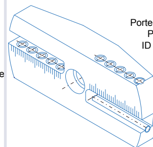
091501031 Porte-outils de la gamme 0° ID 12 - OD 44,5 mm
