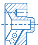
091502824 Porte-outils de la gamme 30° ID 12 - OD 45 mm
