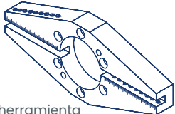
Porta herramienta para mandril tamaño 1 ID 100 - OD 330 mm Item 091506031
