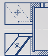
Porta cuchilla 30° ID 16 - OD 50 mm Item 091501101
