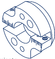
Porta herramienta para mandril tamaño 1 ID 25 - OD 84 mm Item 091502144
