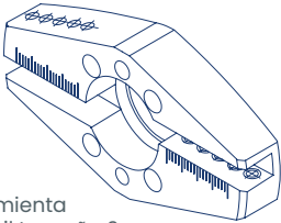
Porta herramienta especial ID 11 - OD 22 mm Item 091505328
