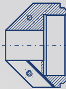
Porta cuchilla 0° ID 25 - OD 66 mm Item 010007079
