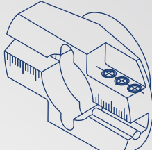
Porta herramienta ID 25 - OD 114,3 mm Item 091503447
