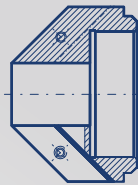
Porta cuchilla 0° ID 25 - OD 66 mm Item 010007079
